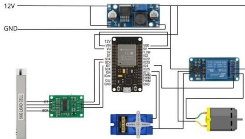
Gambar 2. Hasil implementasi antarmuka perangkat keras.
