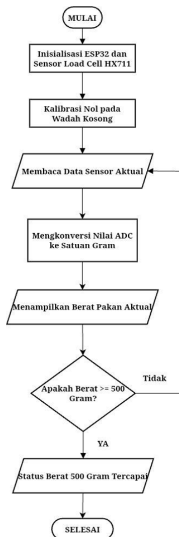
Gambar 5. Desain B3.001 Alur Monitoring berat pakan
