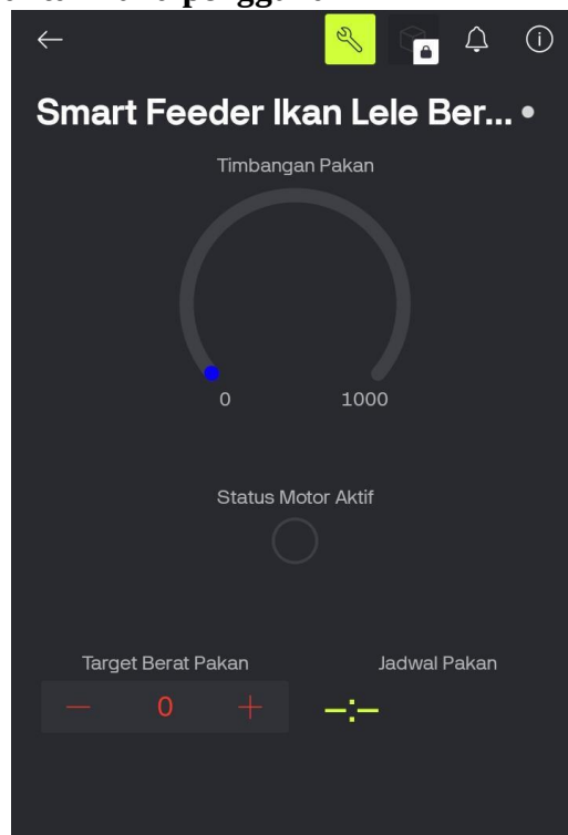
Gambar 4. Hasil implementasi antarmuka pengguna.
